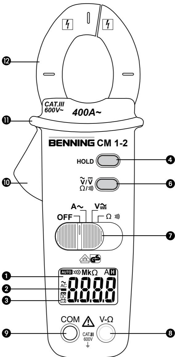
Bild 1b: Gerätefrontseite Fig. 1b: Front tester panel Fig. 1b: Panneau avant de l'appareil Fig. 1b: Parte frontal del equipo obr. 1b: Přední strana přístroje σχήμα 1b: Μπροστινή όψη ill. 1b: Lato anteriore apparecchio
